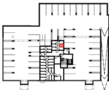
Übersicht Kellergeschoß
